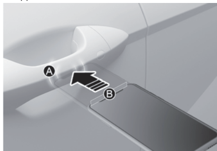
[A] Podloga za autentikaciju na kvaki vozila [B] NFC antena
